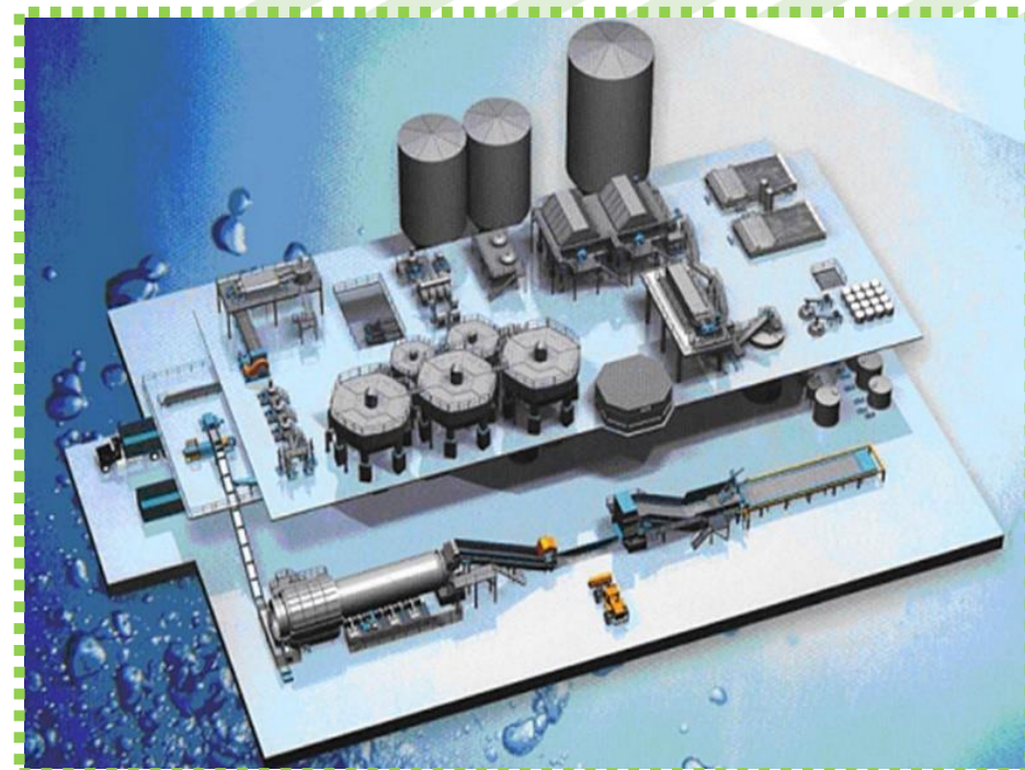
Модель макулатурной линии
