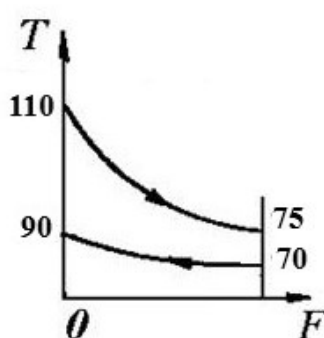
б) противоток
